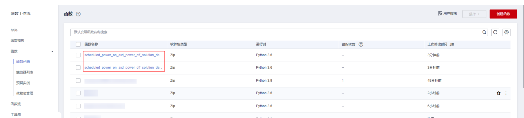
图 3-26 创建的函数
