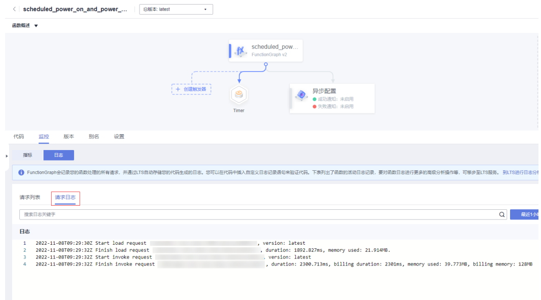
图 3-30 请求日志
