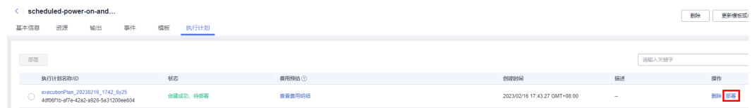
图 3-23 执行计划
